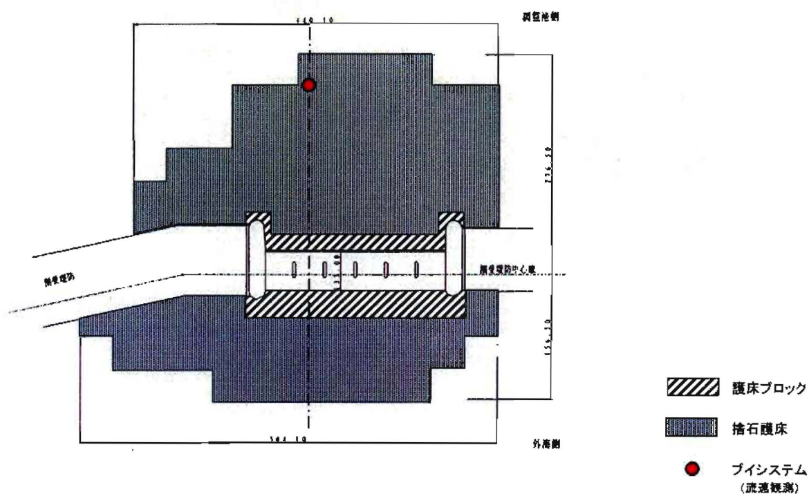
北部排水門 水質観測ブイシステム位置図
